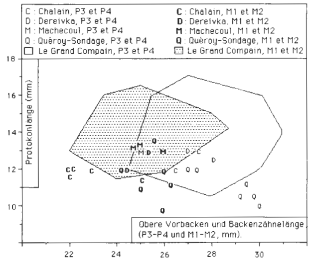
Abb. 5: Variationsbereich der Lngenmae der Abkautungsflche und des Protokons der oberen Backenzhne der Pferde aus Chalain im Vergleich zu denen aus dem Magdalenischen Lagerplatz »Le Grand Compain« (Frankreich) und aus verschiedenen anderen Fundpltzen.
