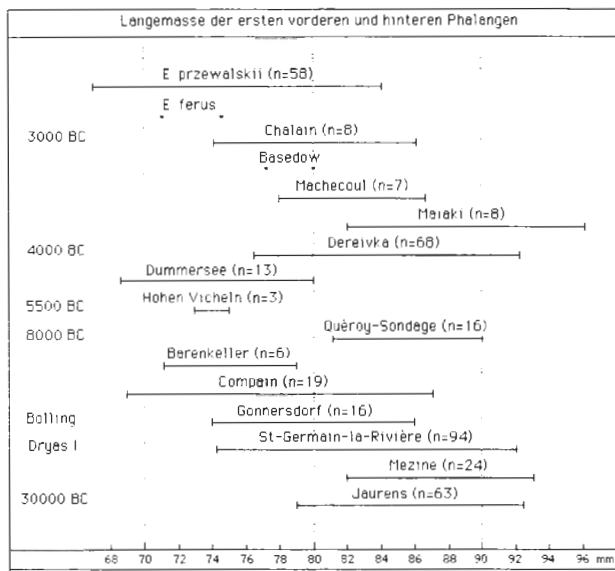
Abb. 4: Variation der Lnge der vorderen und hinteren Fesselbeine verschiedener fossiler und aktueller Pferde.
