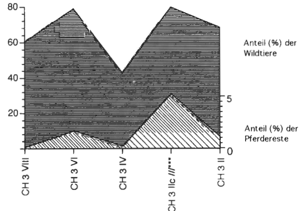
Abb. 7: Variation des Anteils der Pferde (gro schraffiert) und der Wildtierknochen (fein schraffiert) in den verschiedenen Wohnschichten der Siedlung Chalain 3.
