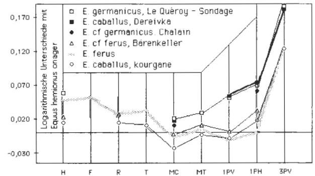
Abb. 6: Ratio-Diagramm der Lngenmae der verschiedenen Skelettpartien und Breitemae der dritten vorderen Phalangen der Pferde aus Chalain im Vergleich zu fossilen und aktuellen Pferden. H= humerus; F= femur; R= radius; T= tibia; MC= dritter Metacarpus; MT= dritter Metatarsus; 1V= erste vordere Phalanx; 1H= erste hintere Phalanx; 3V= dritte vordere Phalanx.
